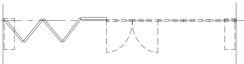
Kanthängd tvåflyglig vikkvägg
