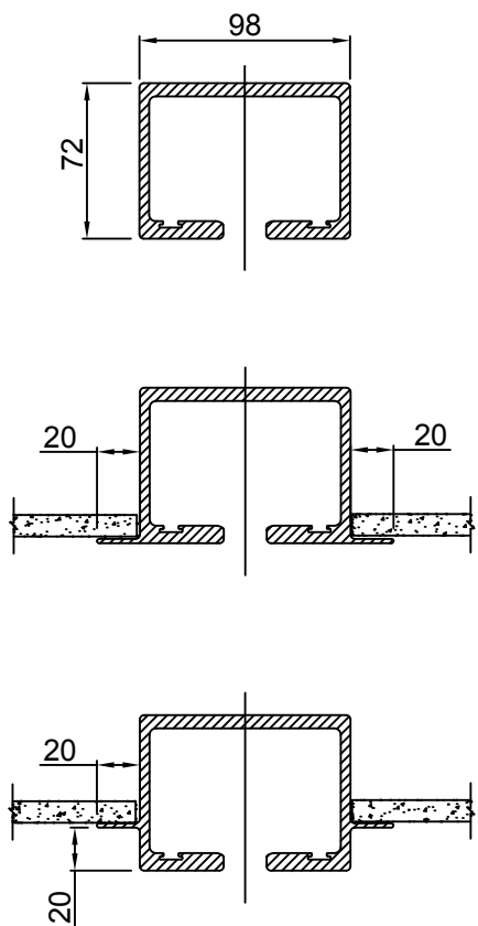
TVÄRSNITT GENOM TAKSKENOR
