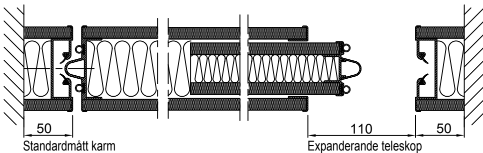
HORISONTELLT SNITT GENOM TELESKOPPANEL OCH VÄGGKARMAR
