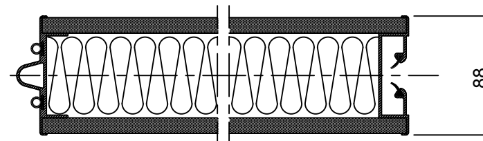
HORISONTELLT SNITT GENOM STANDARDELEMENT
