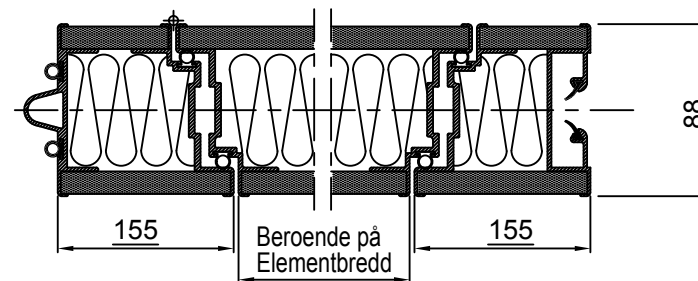
HORISONTELLT SNITT GENOM DÖRRELEMENT
